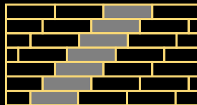
ЛОЖКОВАЯ ДИАГОНАЛЬНАЯ СО СДВИГОМ В ЧЕТВЕРТЬ КИРПИЧА
